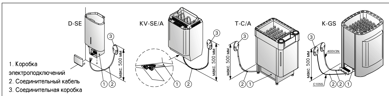
Рисунок 8. Установка каменки
