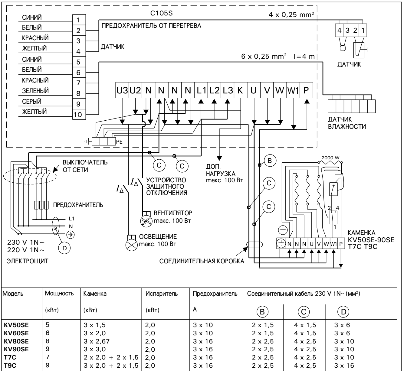
Рисунок 12. 1-Фазная сеть
